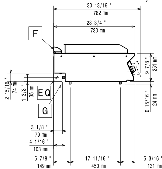
Zij aanzicht
